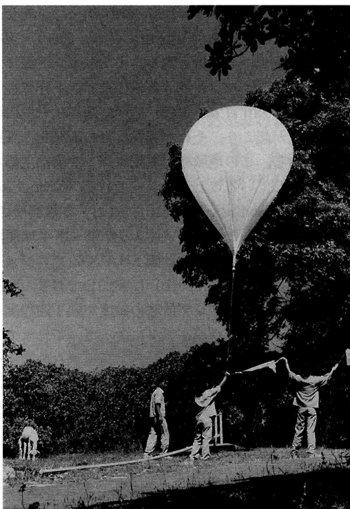
第1図 ワトゥコセック観測所におけるオゾンゾンデ観測 (1995年5月)。
