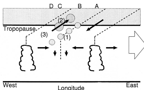
第5図 オゾン輸送を引き起こした東進する擾乱システムの経度高度概念図。点線は東西風ゼロの位置を示す。オゾン増大域を影をつけた円で示す。A~Dは、この擾乱が観測点を通過した日にちを示す。すなわち、A: 5月6~11日、B: 5月15~16日、C: 5月21~22日、D: 5月26日。オゾン輸送過程はそれぞれ(1)赤道ケルビン波とMJOに伴う下降流による輸送、(2)赤道ケルビン波の碎波位相部(西風極大)における大気混合、(3)水平混合による対流圏への不可逆輸送。Fujiwara et al. (1998a) より引用。
